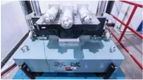
Shock Test Bench / 冲击试验台
